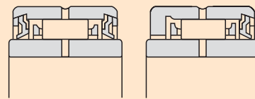
Fig. 6 Series NA49..L(LL)
